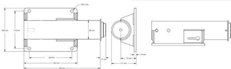
Tuotenumeron 5BW5 mitat
