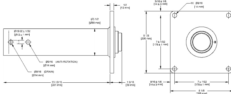
Tuotenumeron 5BF5 mitat
